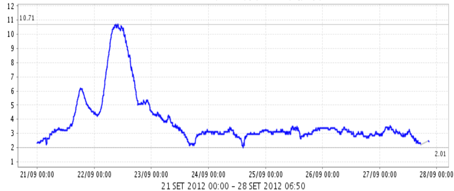
Rio Corumbataí - Batovi (D4-043) / (4D-018T) Q(m 3 /s)
