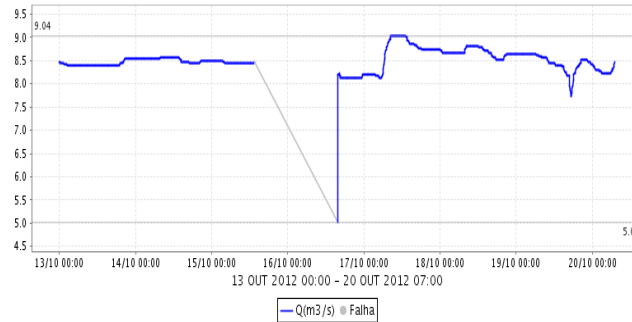
Rio Atibaia em Atibaia (E3-111T / 3E-063T) Q(m 3 /s)
