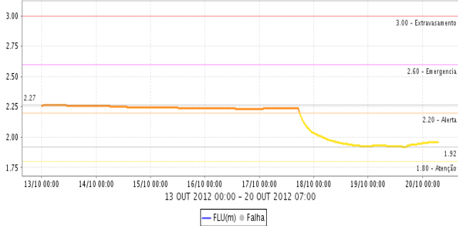
R. Cachoeira Captação Piracaja(E3-110T/3E-116T) FLU(m)
