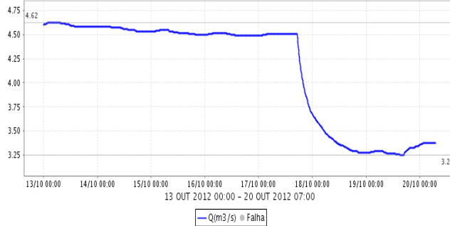
R. Cachoeira Captação Piracaja(E3-110T/3E-116T) Q(m 3 /s)
