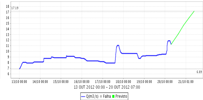
Rio Camanduacaia em Dal Bo (D3-044T / 3D-001T) Q(m³/s)
