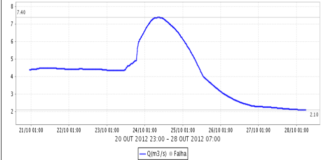
Rio Atibaia em Atibaia (E3-111T / 3E-063T) Q(m3/s)
