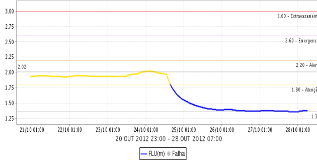
R. Cachoeira Captação Piracala(E3-110T/3E-116T) FLU(m)
