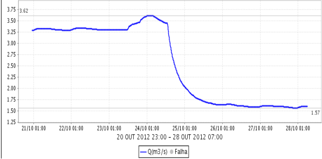
R. Cachoeira Captação Piracala(E3-110T/3E-116T) Q(m3/s)
