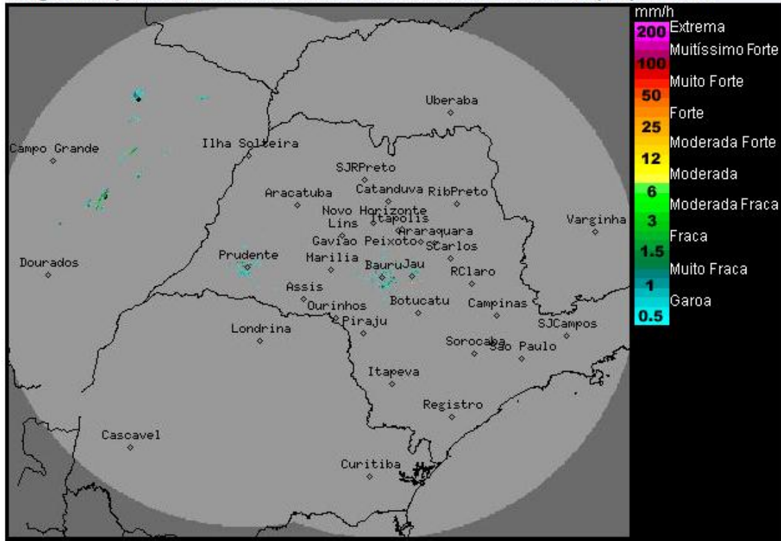
Imagem Composta dos Radares de Bauru e de Presidente Prudente - 22/11/12 13:00
