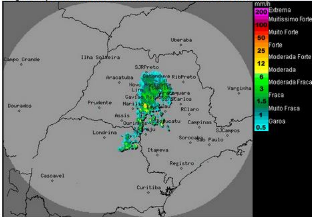
Imagem Composta dos Radares de Bauru e de Presidente Prudente - 23/01/14 10:00
