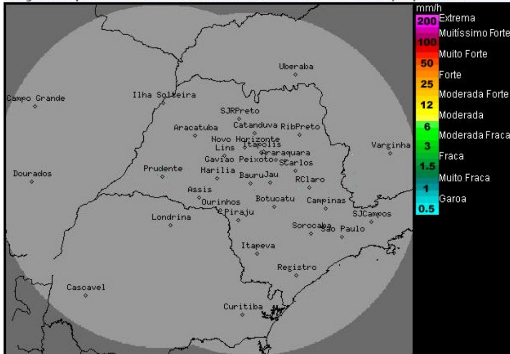
Imagem Composta dos Radares de Bauru e de Presidente Prudente - 29/01/14 10:15
