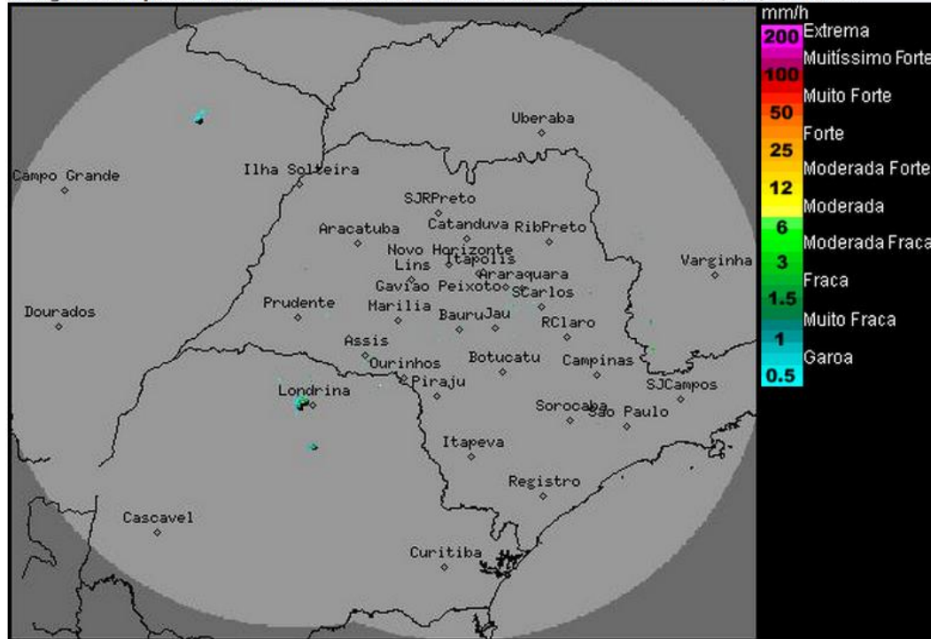
Imagem Composta dos Radares de Bauru e de Presidente Prudente - 30/01/14 10:15
