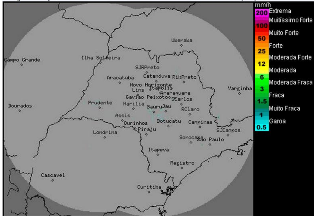
Imagem Composta dos Radares de Bauru e de Presidente Prudente - 14/03/2014 10:45
