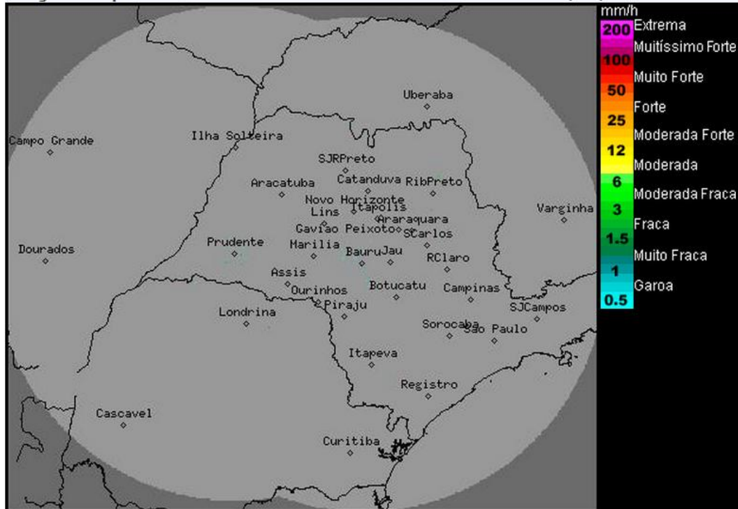
Imagem Composta dos Radares de Bauru e de Presidente Prudente - 30/06/2014 11:00
