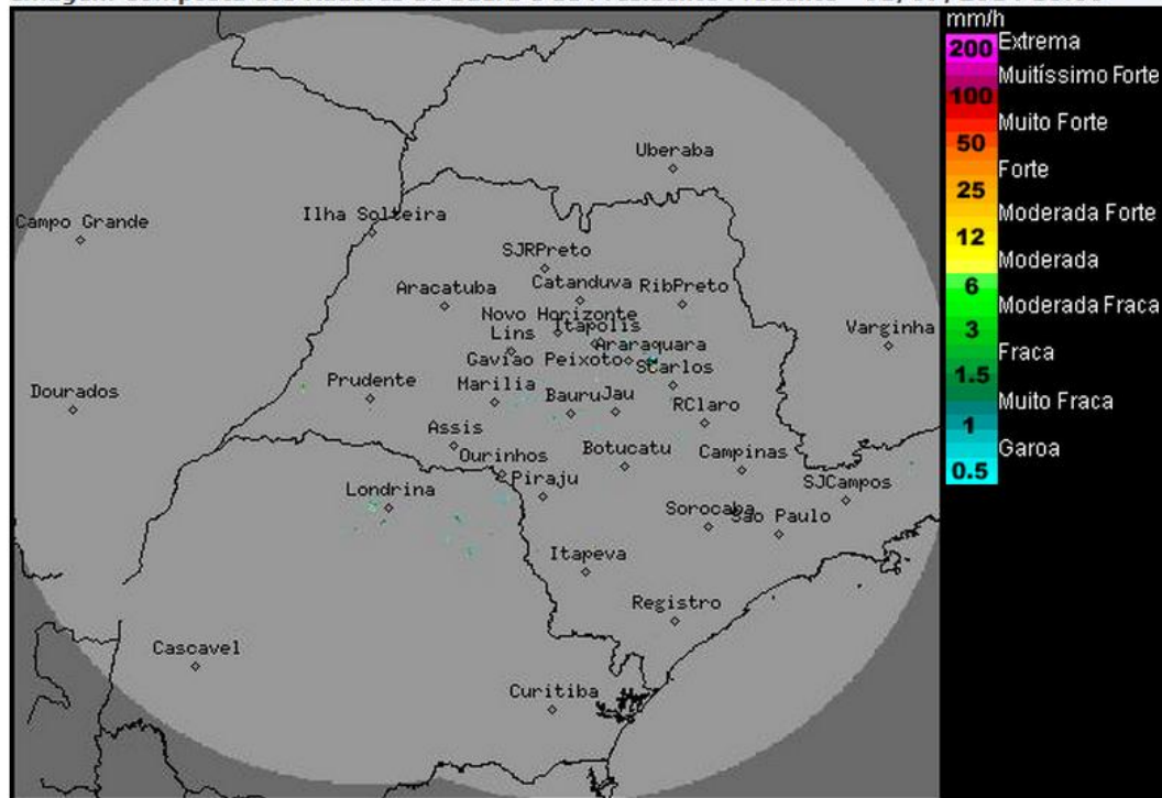
Imagem Composta dos Radares de Bauru e de Presidente Prudente - 01/07/2014 10:00
