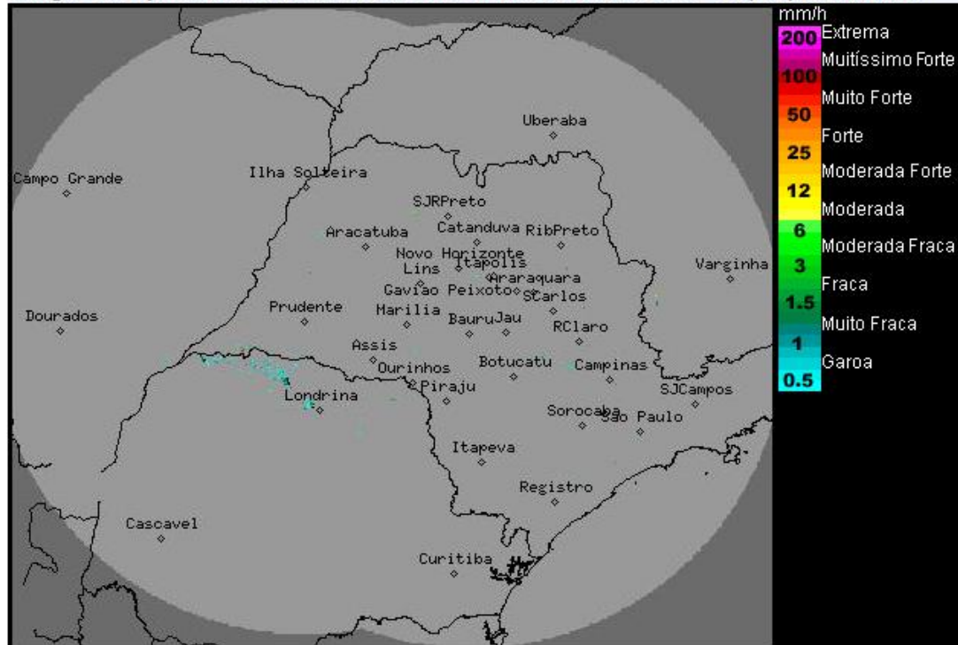
Imagem Composta dos Radares de Bauru e de Presidente Prudente - 13/10/2014 09:00
