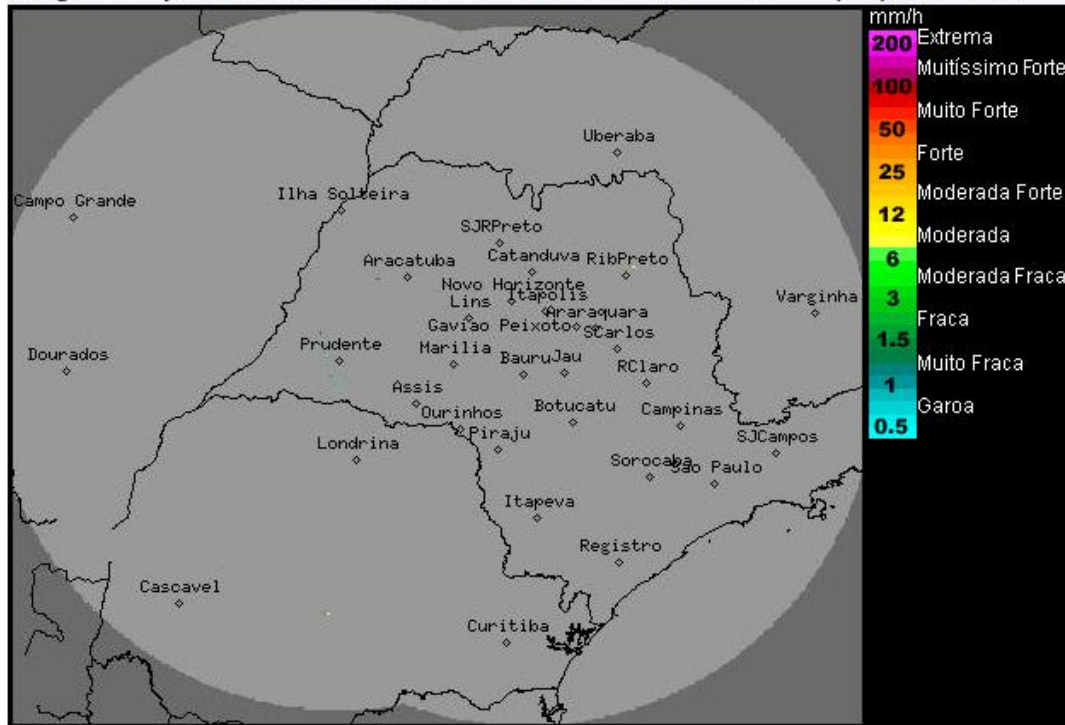
Imagem Composta dos Radares de Bauru e de Presidente Prudente - 15/10/2014 09:00
