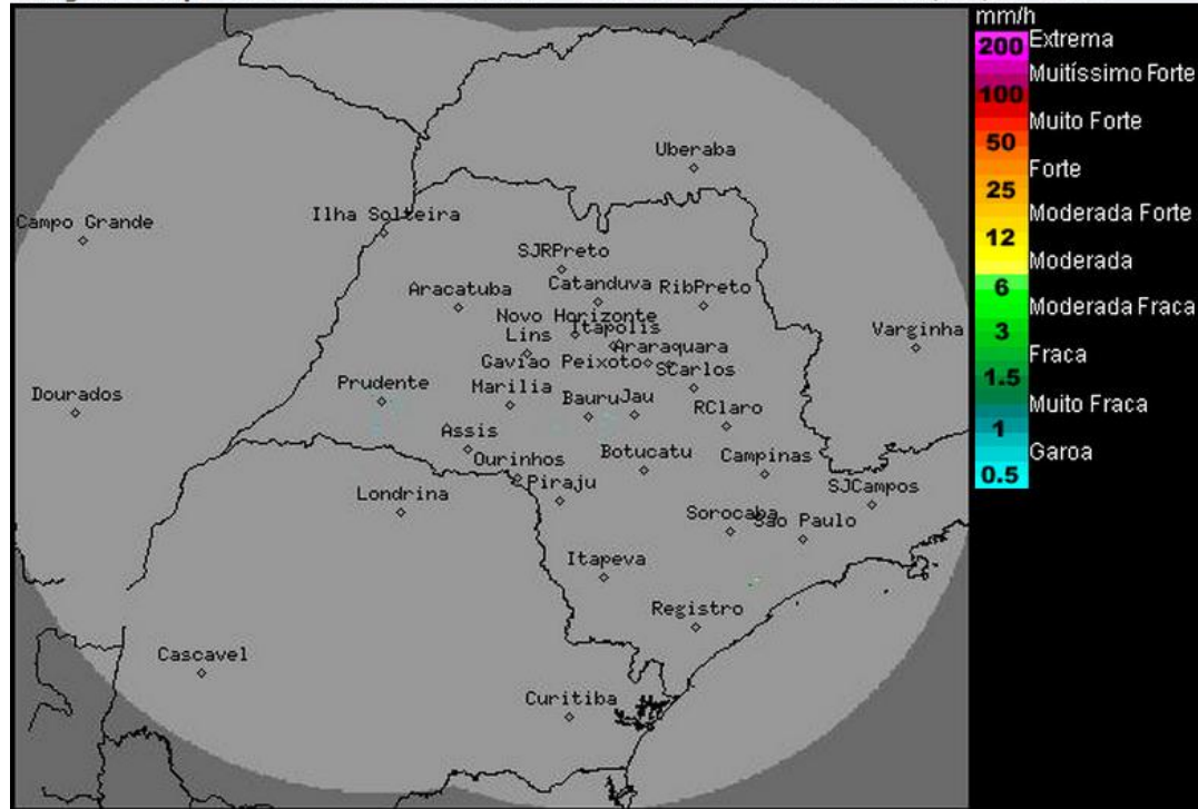
Imagem Composta dos Radares de Bauru e de Presidente Prudente - 27/10/14 13:00
