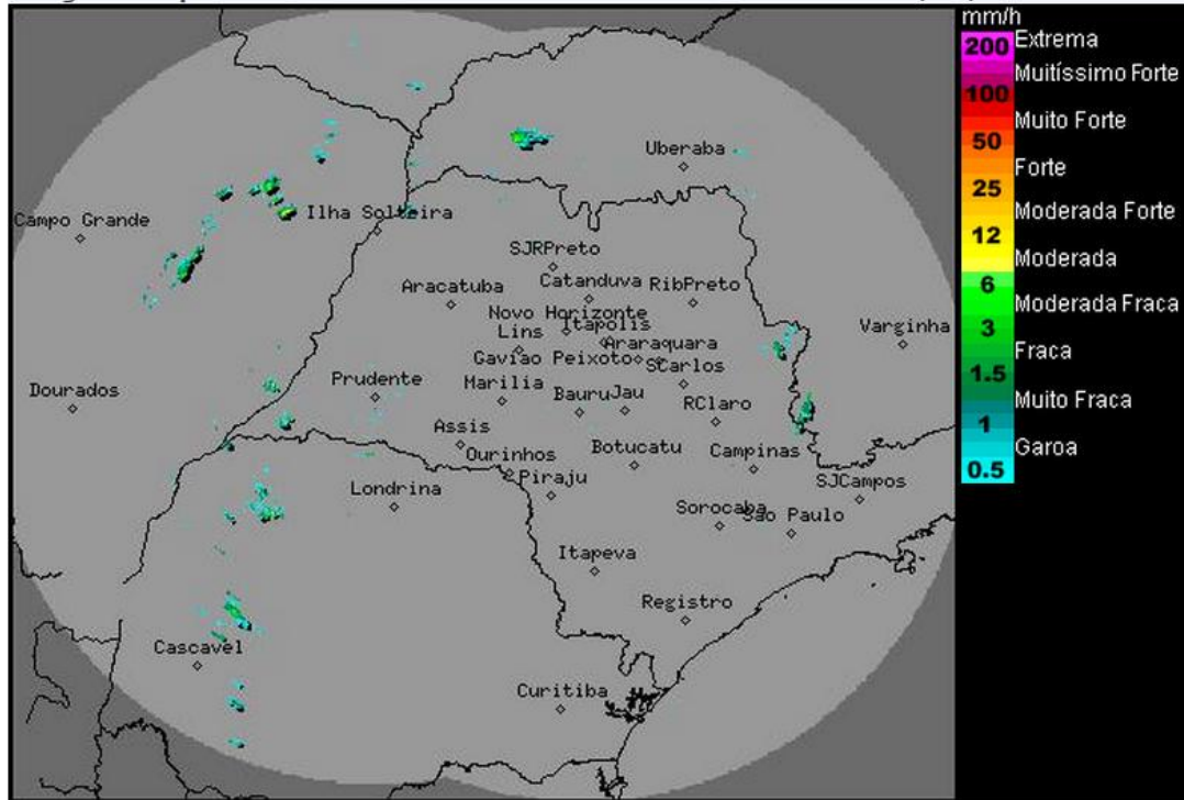
Imagem Composta dos Radares de Bauru e de Presidente Prudente - 30/10/14 12:45
