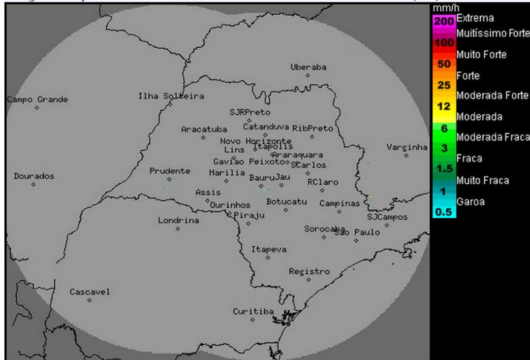
Imagem Composta dos Radares de Bauru e de Presidente Prudente - 06/11/14 10:45
