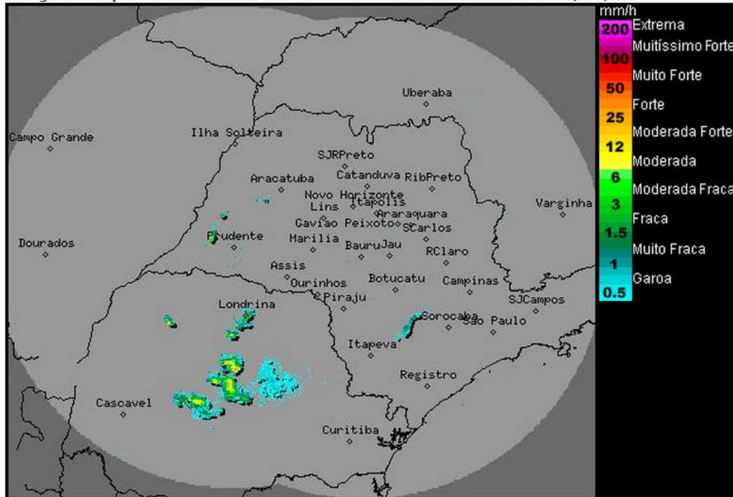
Imagem Composta dos Radares de Bauru e de Presidente Prudente - 07/11/14 10:45
