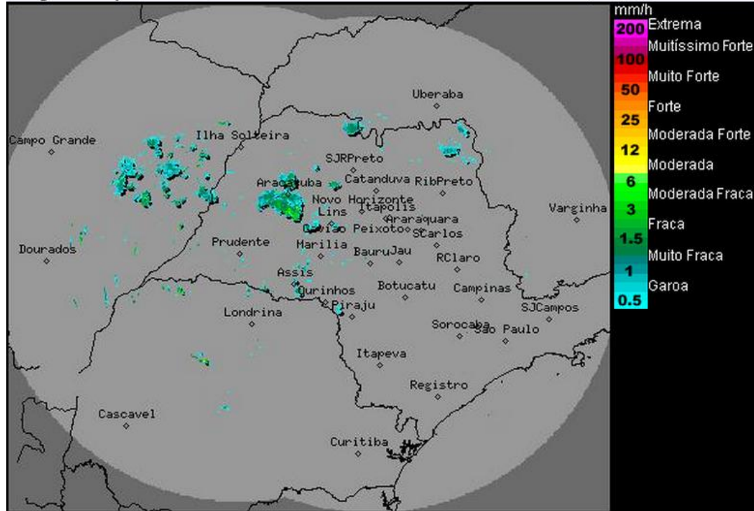
Imagem Composta dos Radares de Bauru e de Presidente Prudente - 25/11/14 11:00
