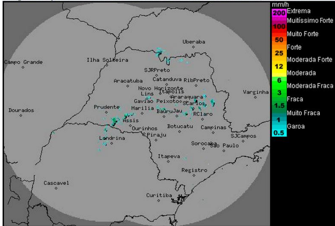
Imagem Composta dos Radares de Bauru e de Presidente Prudente - 26/11/14 10:00
