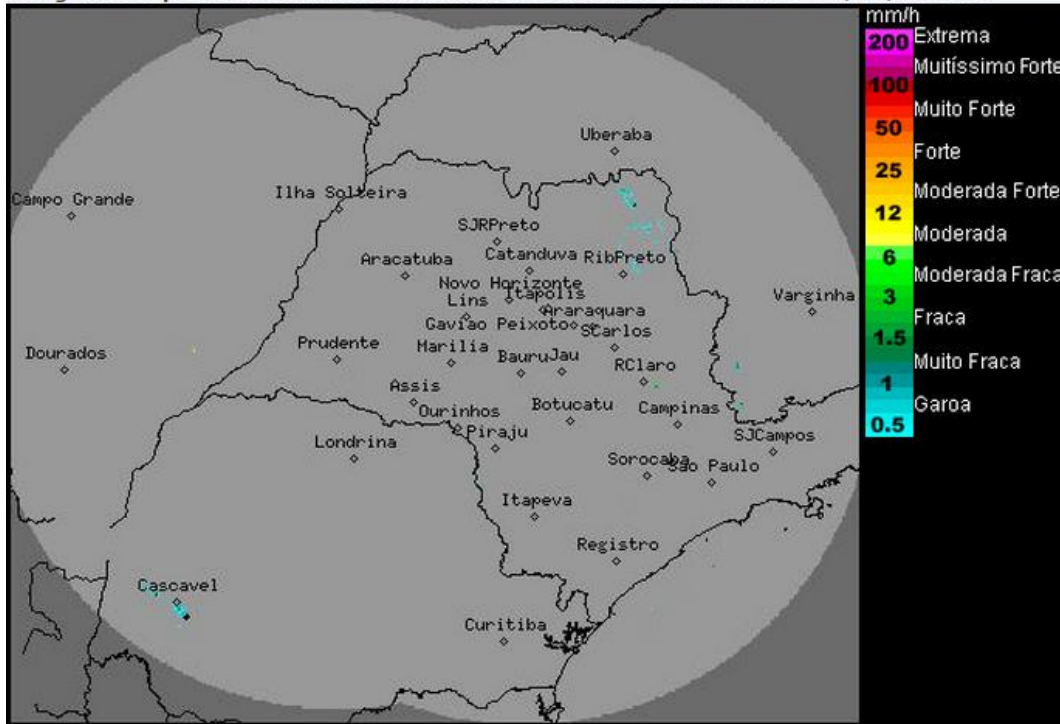
Imagem Composta dos Radares de Bauru e de Presidente Prudente - 31/12/14 10:45
