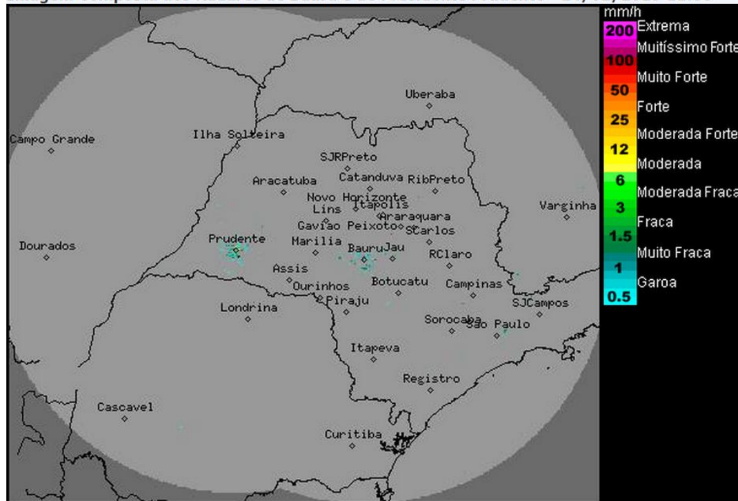
Imagem Composta dos Radares de Bauru e de Presidente Prudente - 24/02/2015 11:00
