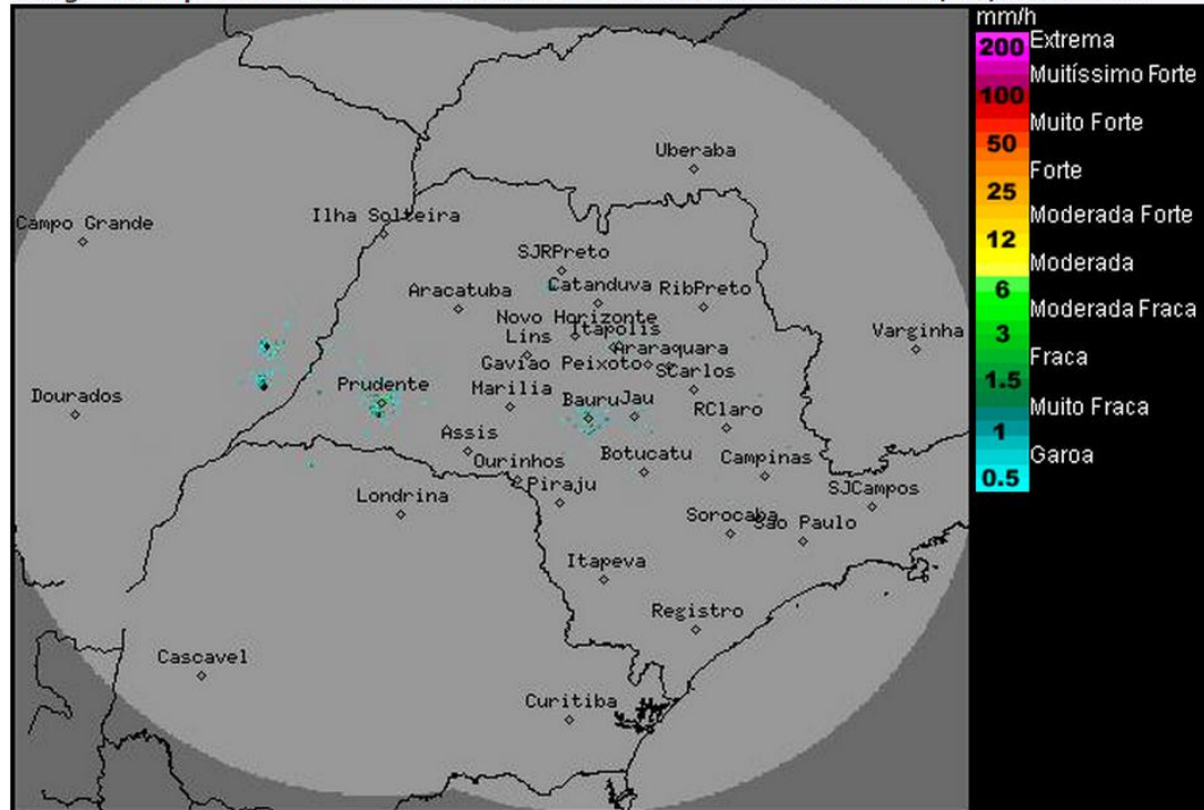
Imagem Composta dos Radares de Bauru e de Presidente Prudente - 01/04/2015 10:00
