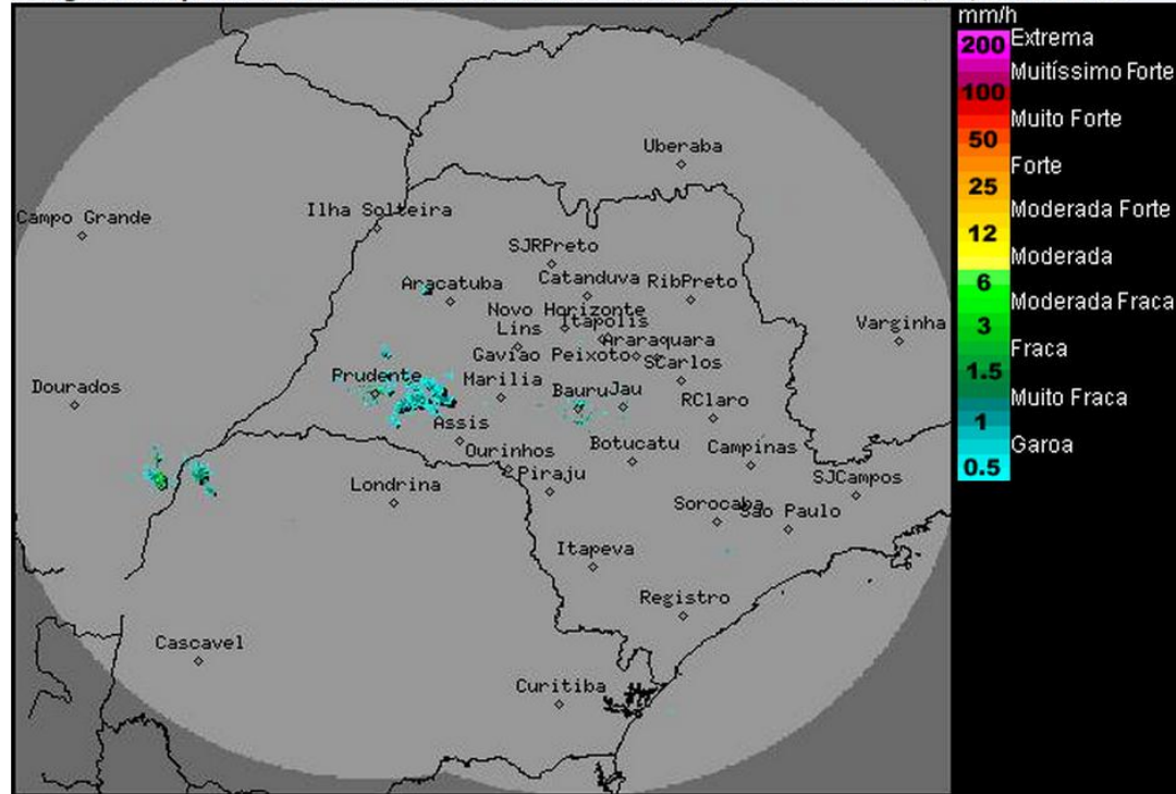
Imagem Composta dos Radares de Bauru e de Presidente Prudente - 14/04/2015 11:00
