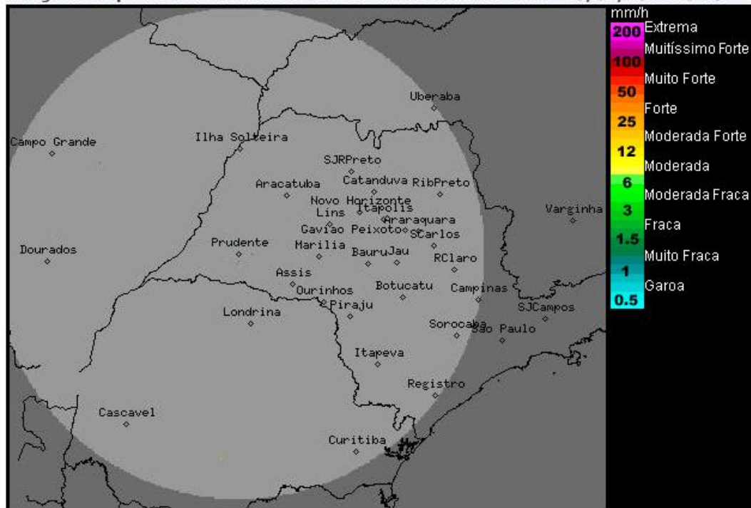
Imagem Composta dos Radares de Bauru e de Presidente Prudente - 30/04/2015 10:30
