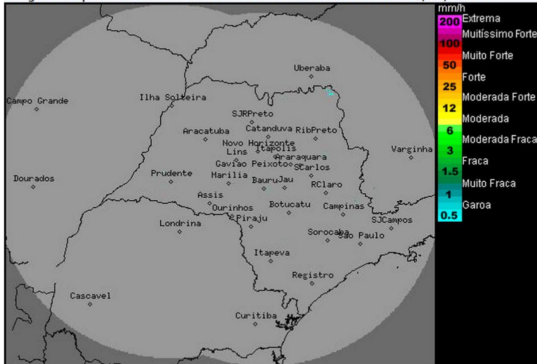
Imagem Composta dos Radares de Bauru e de Presidente Prudente - 06/05/2015 10:00
