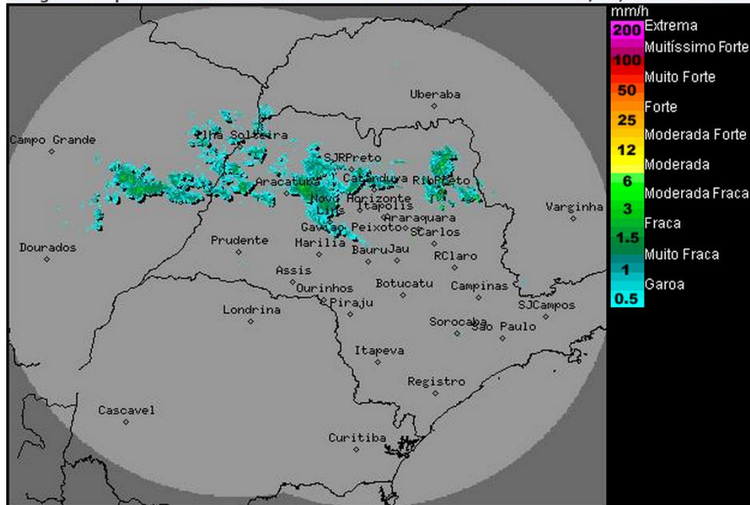
Imagem Composta dos Radares de Bauru e de Presidente Prudente - 02/06/2015 11:15
