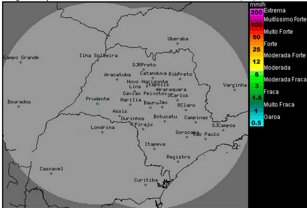
Imagem Composta dos Radares de Bauru e de Presidente Prudente - 10/06/2015 11:00
