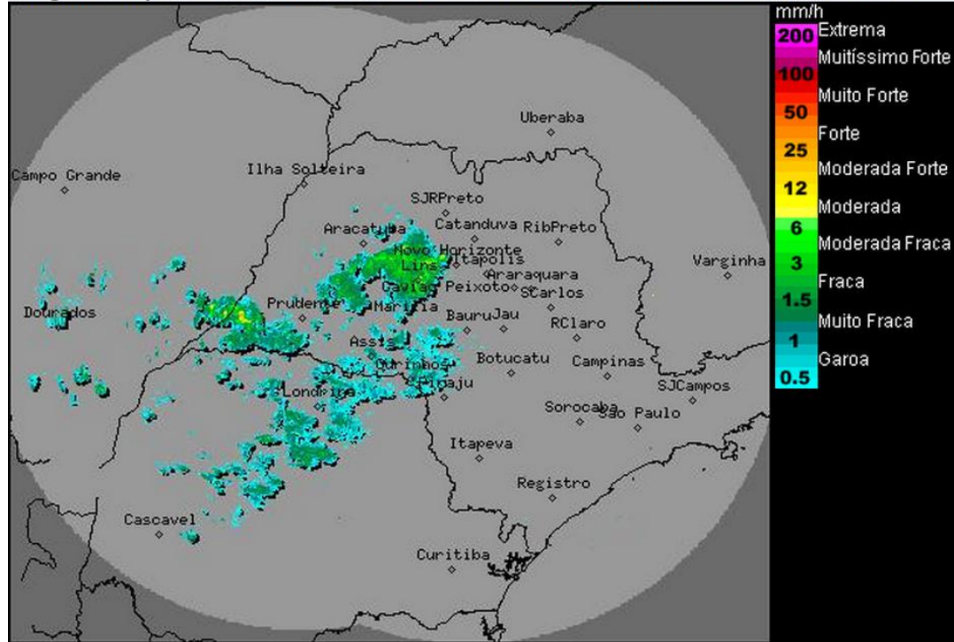
Imagem Composta dos Radares de Bauru e de Presidente Prudente - 02/07/2015 11:30
