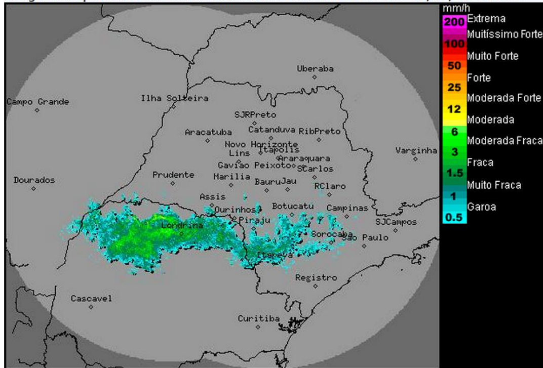
Imagem Composta dos Radares de Bauru e de Presidente Prudente - 03/07/2015 10:45
