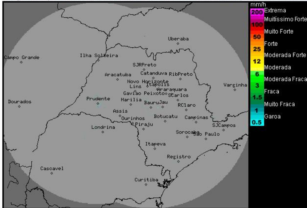
Imagem Composta dos Radares de Bauru e de Presidente Prudente - 04/08/2015 11:45
