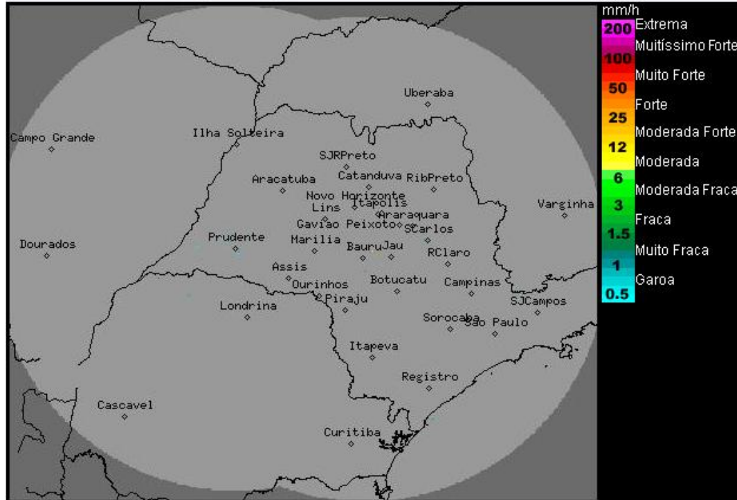
Imagem Composta dos Radares de Bauru e de Presidente Prudente - 13/08/2015 11:30
