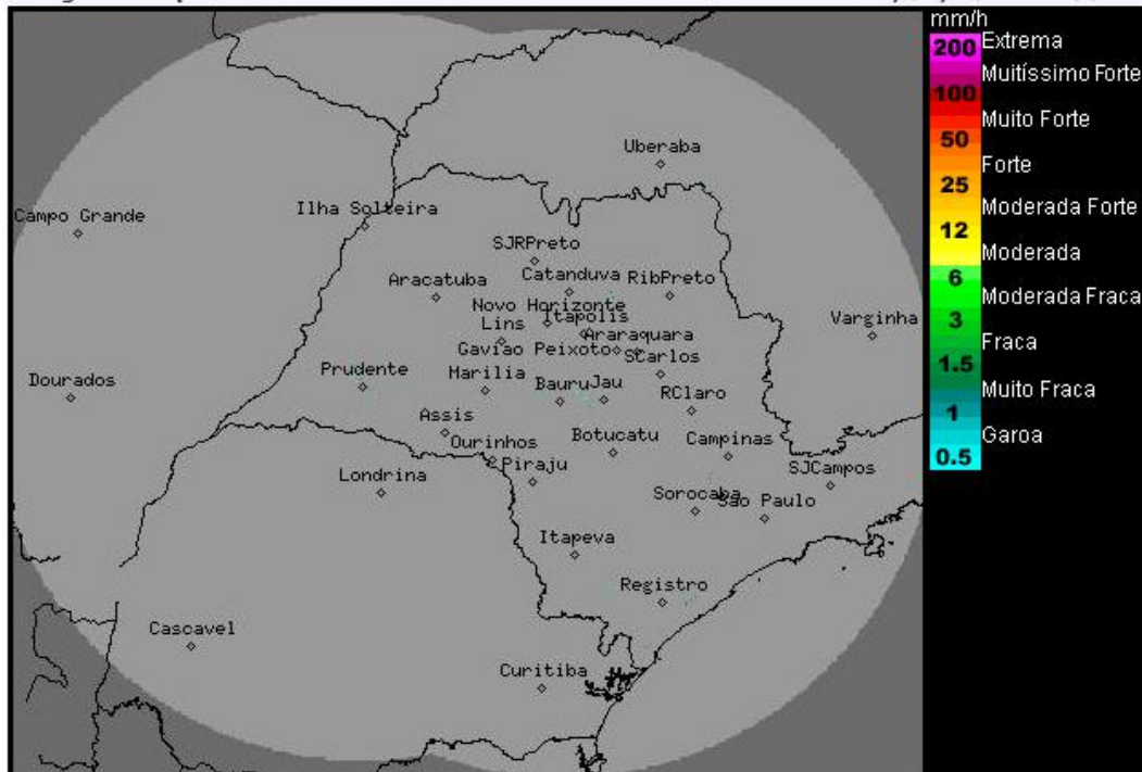
Imagem Composta dos Radares de Bauru e de Presidente Prudente - 14/08/2015 12:00
