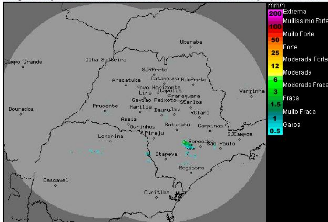
Imagem Composta dos Radares de Bauru e de Presidente Prudente - 04/09/2015 12:30
