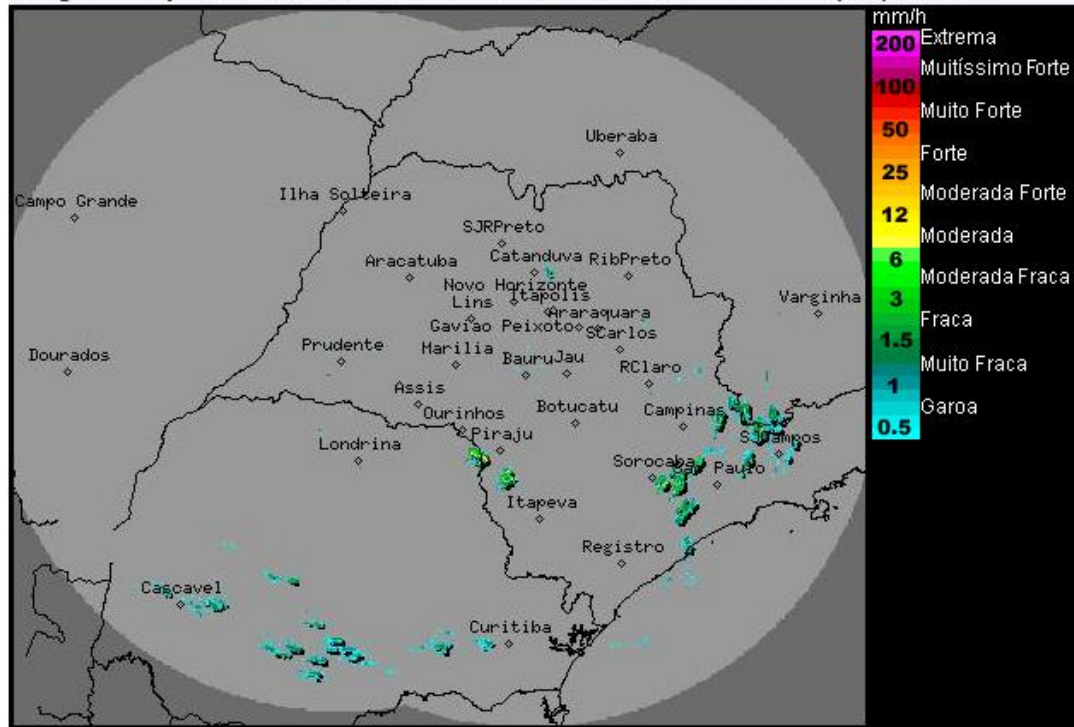
Imagem Composta dos Radares de Bauru e de Presidente Prudente - 22/10/15 11:45
