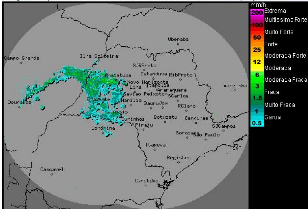
Imagem Composta dos Radares de Bauru e de Presidente Prudente - 23/10/15 11:15
