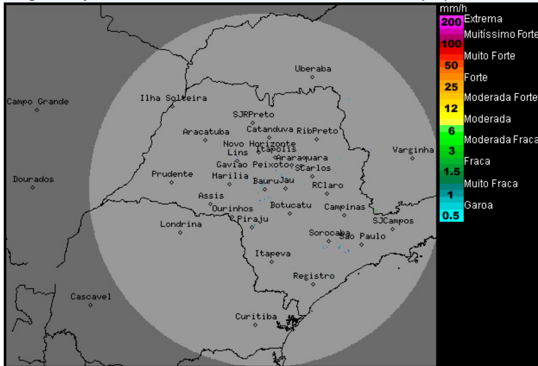
Imagem Composta dos Radares de Bauru e de Presidente Prudente - 13/11/15 11:30
