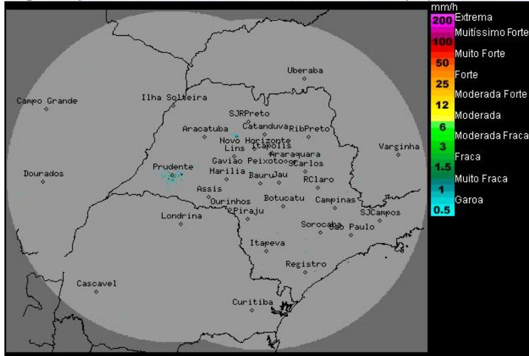
Imagem Composta dos Radares de Bauru e de Presidente Prudente - 14/07/2016 14:00
