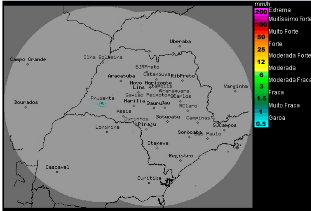
Imagem Composta dos Radares de Bauru e de Presidente Prudente - 22/08/2016 12:00
