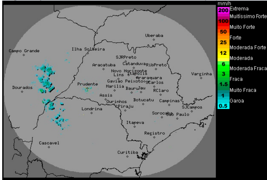
Imagem Composta dos Radares de Bauru e de Presidente Prudente - 29/08/2016 12:45
