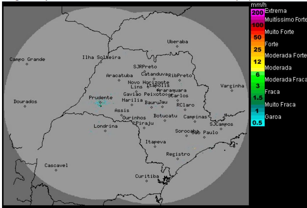
Imagem Composta dos Radares de Bauru e de Presidente Prudente - 23/09/2016 12:00
