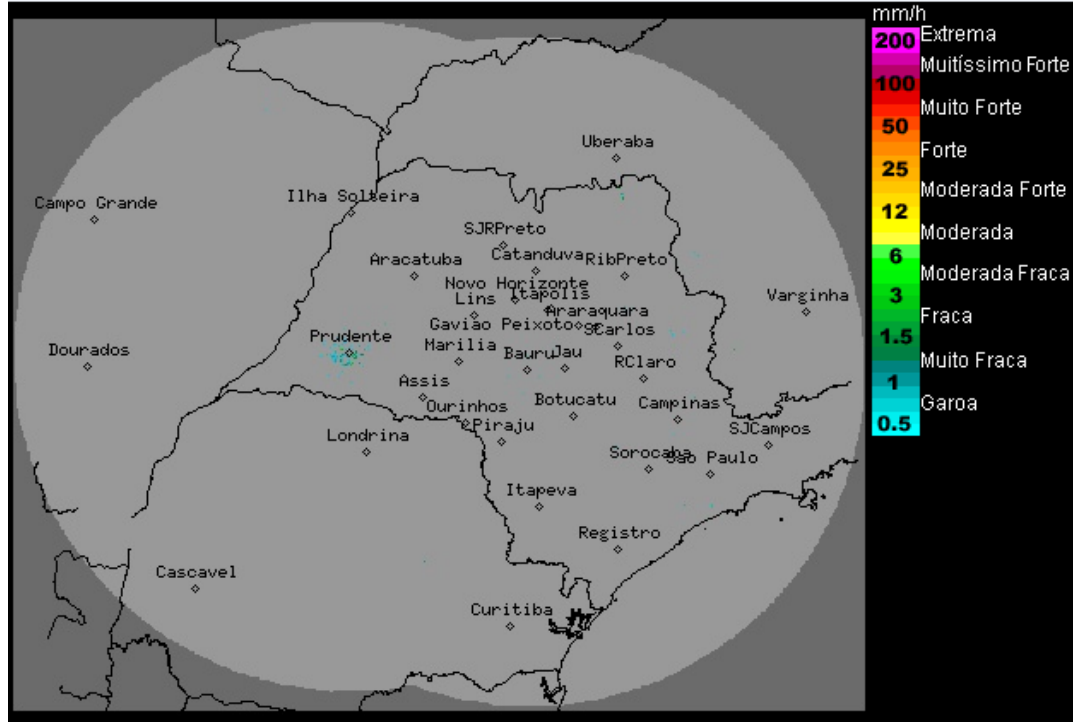
Imagem Composta dos Radares de Bauru e de Presidente Prudente - 27/09/2016 11:00
