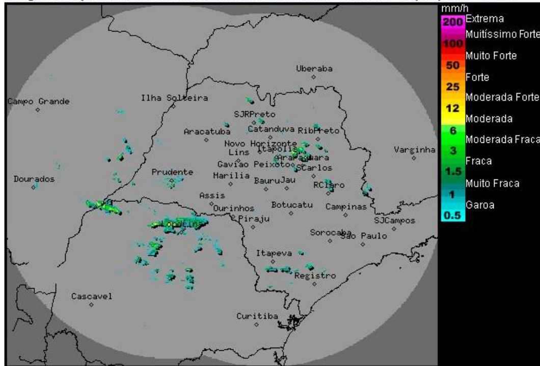
Imagem Composta dos Radares de Bauru e de Presidente Prudente - 11/10/2016 13:00
