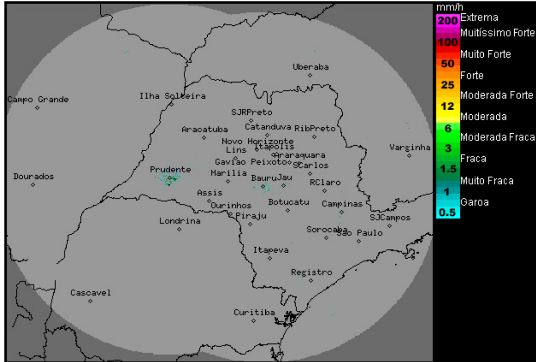
Imagem Composta dos Radares de Bauru e de Presidente Prudente - 29/12/16 11:00
