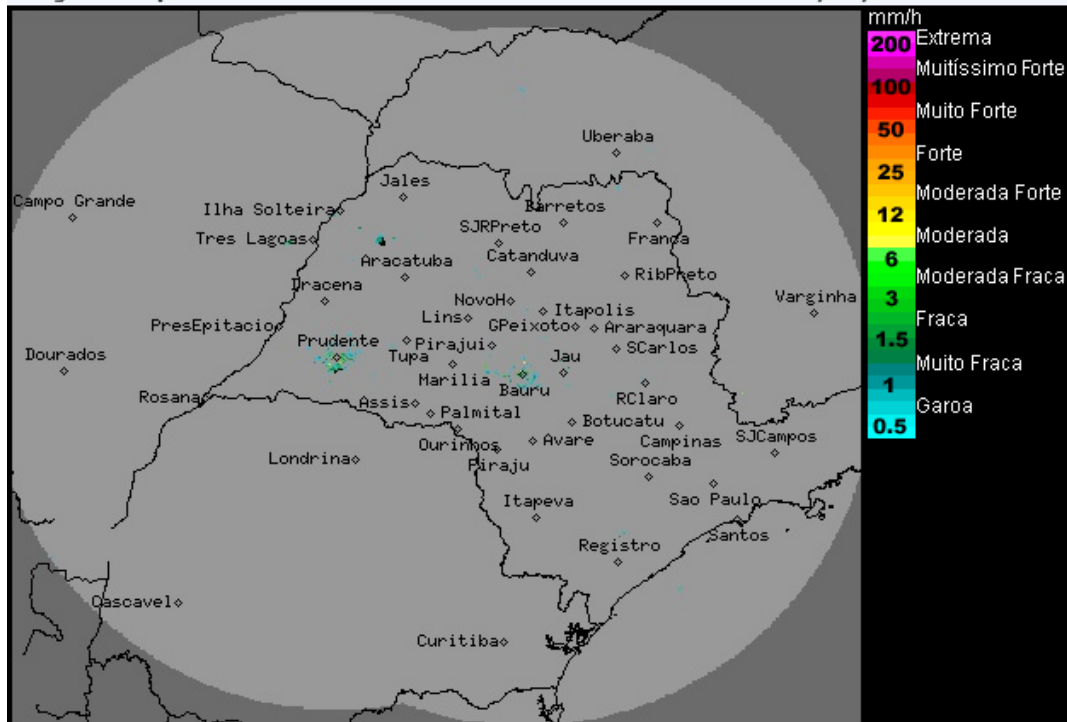
Imagem Composta dos Radares de Bauru e de Presidente Prudente - 12/04/2017 10:15
