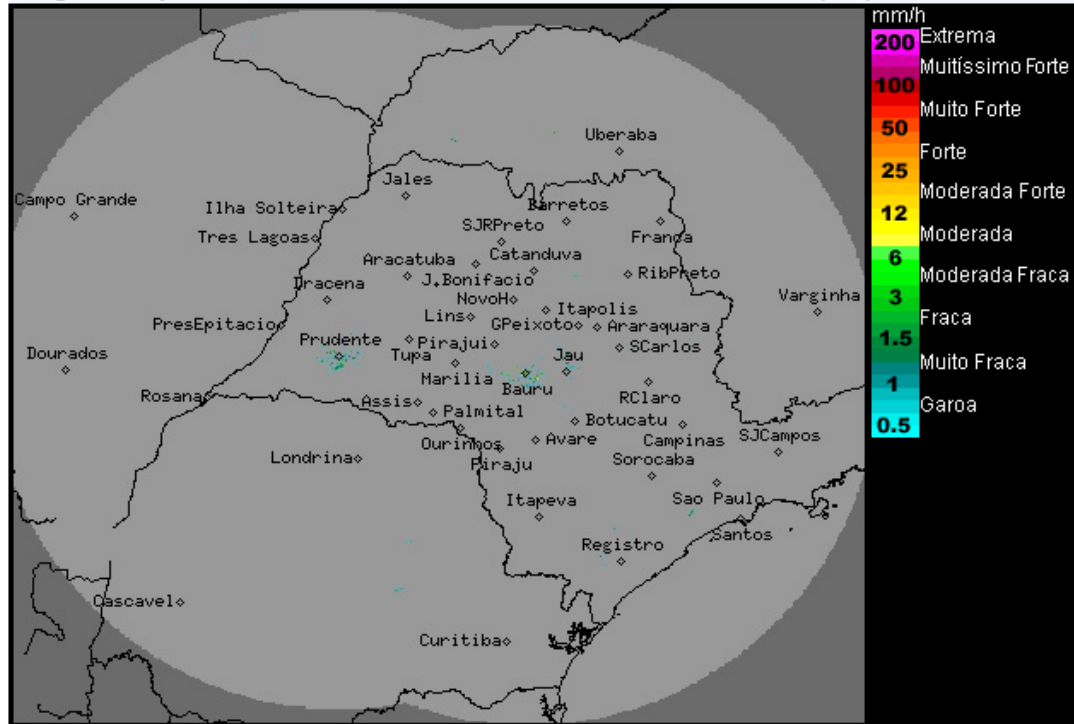
Imagem Composta dos Radares de Bauru e de Presidente Prudente - 11/05/2017 09:00
