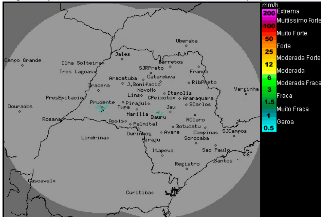
Imagem Composta dos Radares de Bauru e de Presidente Prudente - 12/05/2017 09:00
