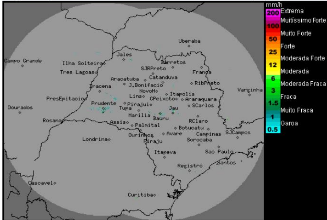
Imagem Composta dos Radares de Bauru e de Presidente Prudente - 30/05/2017 09:00
