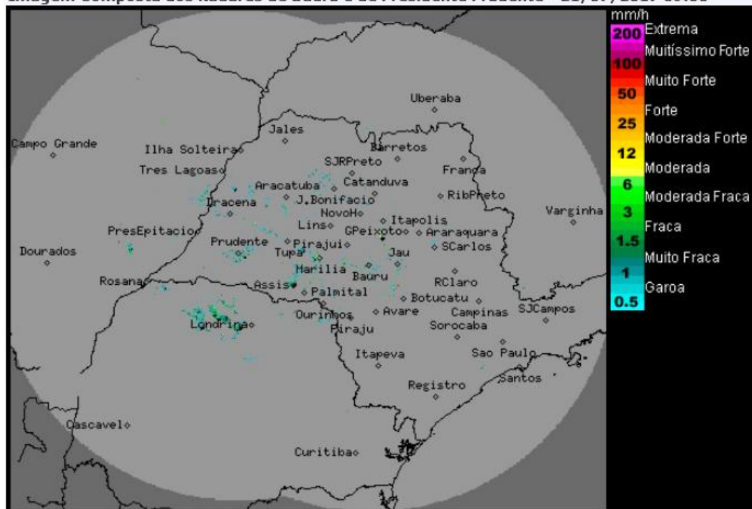
Imagem Composta dos Radares de Bauru e de Presidente Prudente - 21/07/2017 09:00
