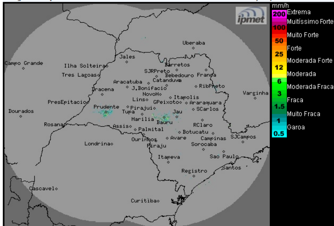
Imagem Composta dos Radares de Bauru e de Presidente Prudente - 12/12/17 09:00
