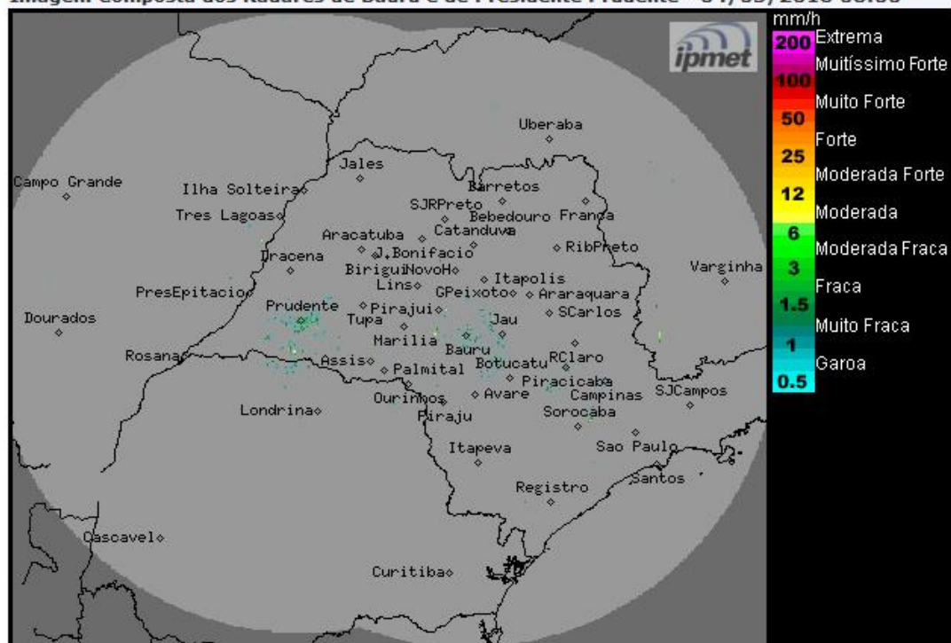
Imagem Composta dos Radares de Bauru e de Presidente Prudente - 04/05/2018 08:00
