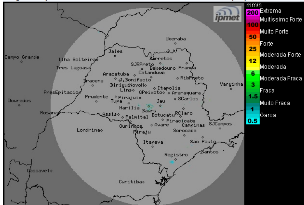
Imagem Composta dos Radares de Bauru e de Presidente Prudente - 08/05/2018 08:15
